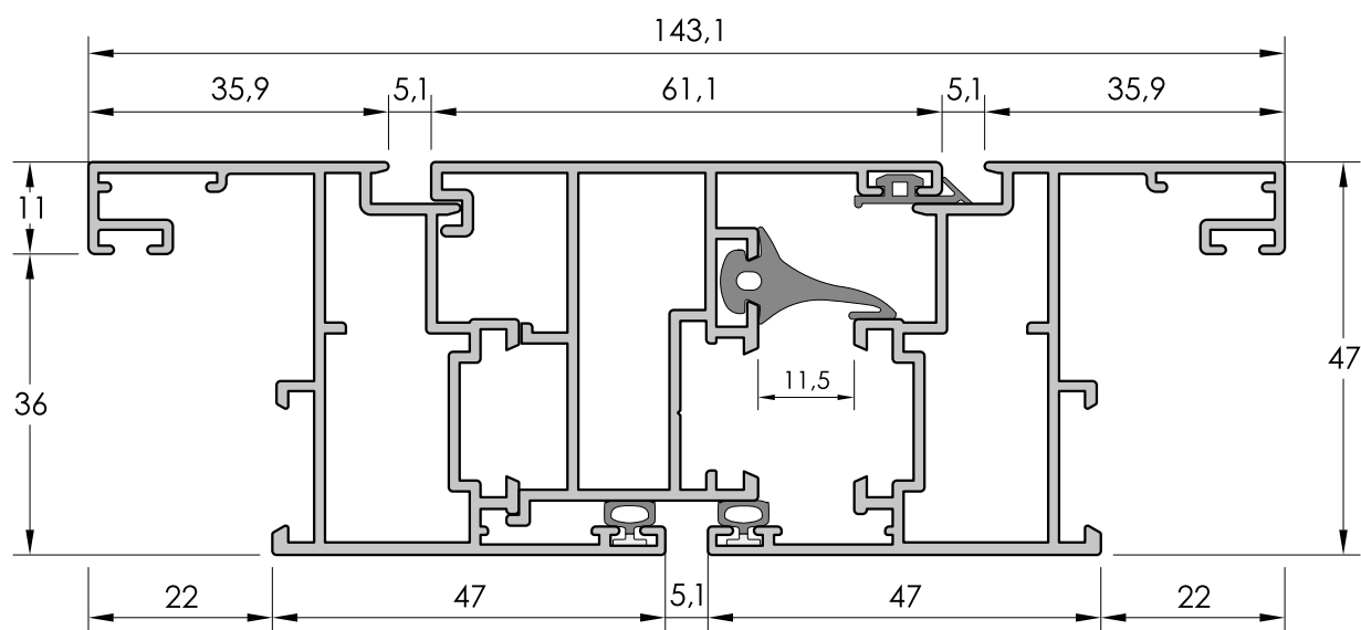
SECCIÓN HORIZONTAL HOJA 35126 - INVERSOR 34133 - HOJA 35126
