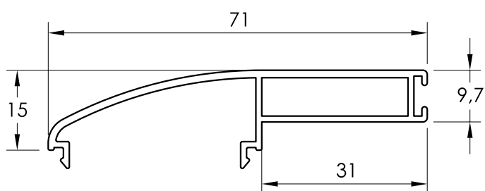
65007 TAPA LATERAL
