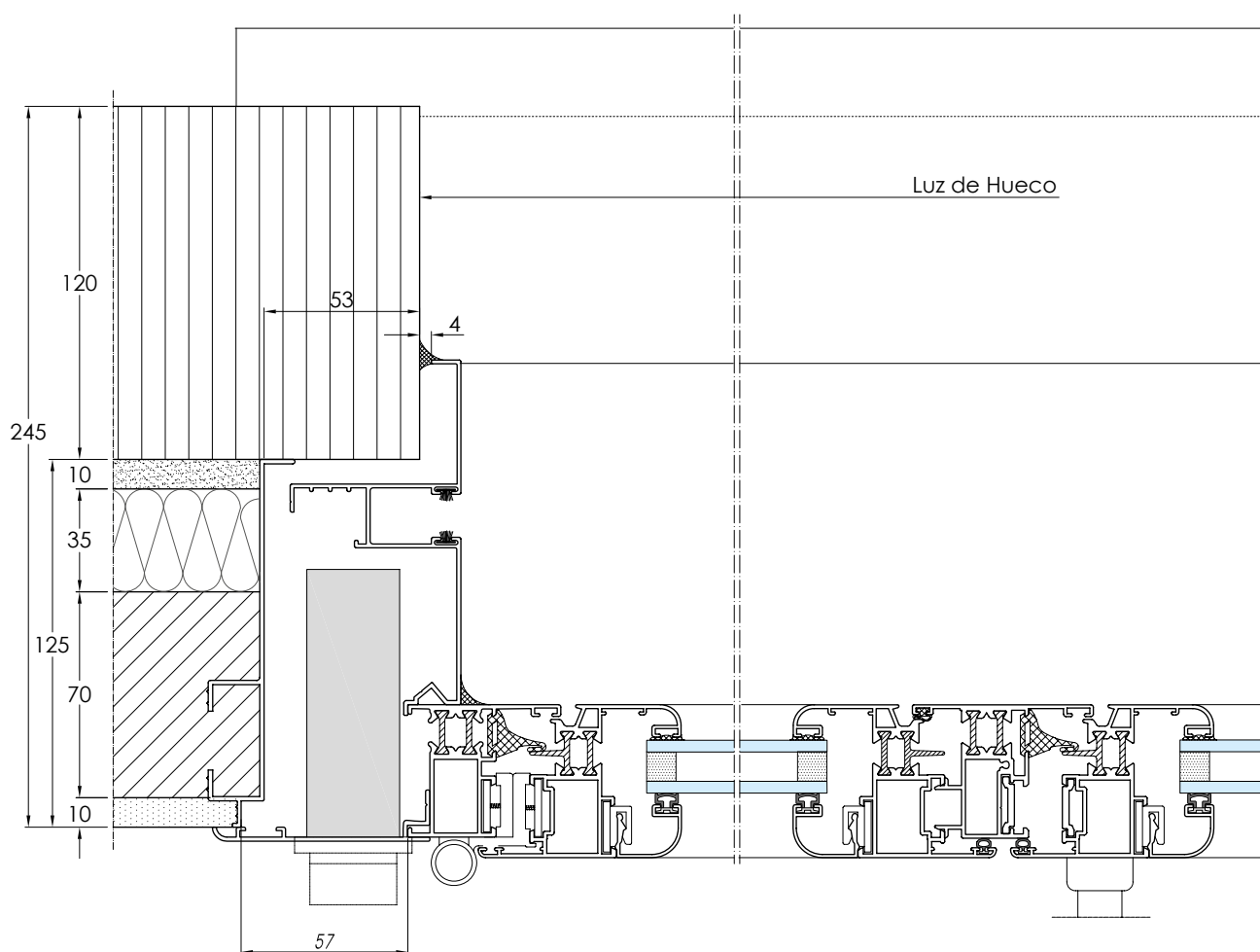
SECCIÓN HORIZONTAL 1-1
