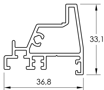
24953 BAJO PUERTA (PASO LIBRE)
