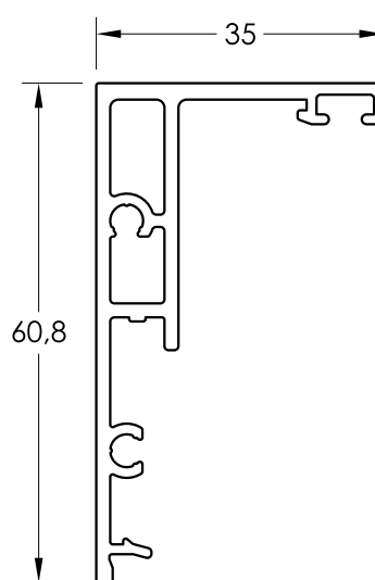
24915 PERFIL DE CRUCE FIJO
