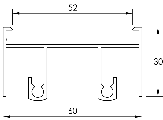
27083 GUÍA SUPERIOR
