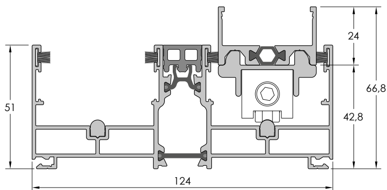
SECCIÓN VERTICAL, NUDO INFERIOR MARCO 2 CARRILES
