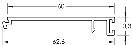
24916 TAPA DE MARCO FIJO
