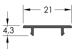
AH 45801 TAPA UMBRAL PARA CERRADEROS
