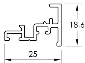
24961 BAJO PUERTA (CON UMBRAL)
