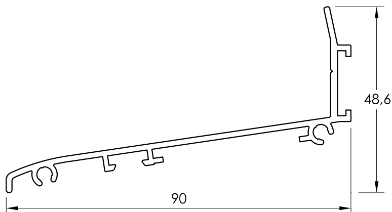
65460 VIERTEAGUAS PARED
