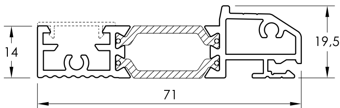
PM 091 UMBRAL IT-71-NG PARA CERRADEROS
