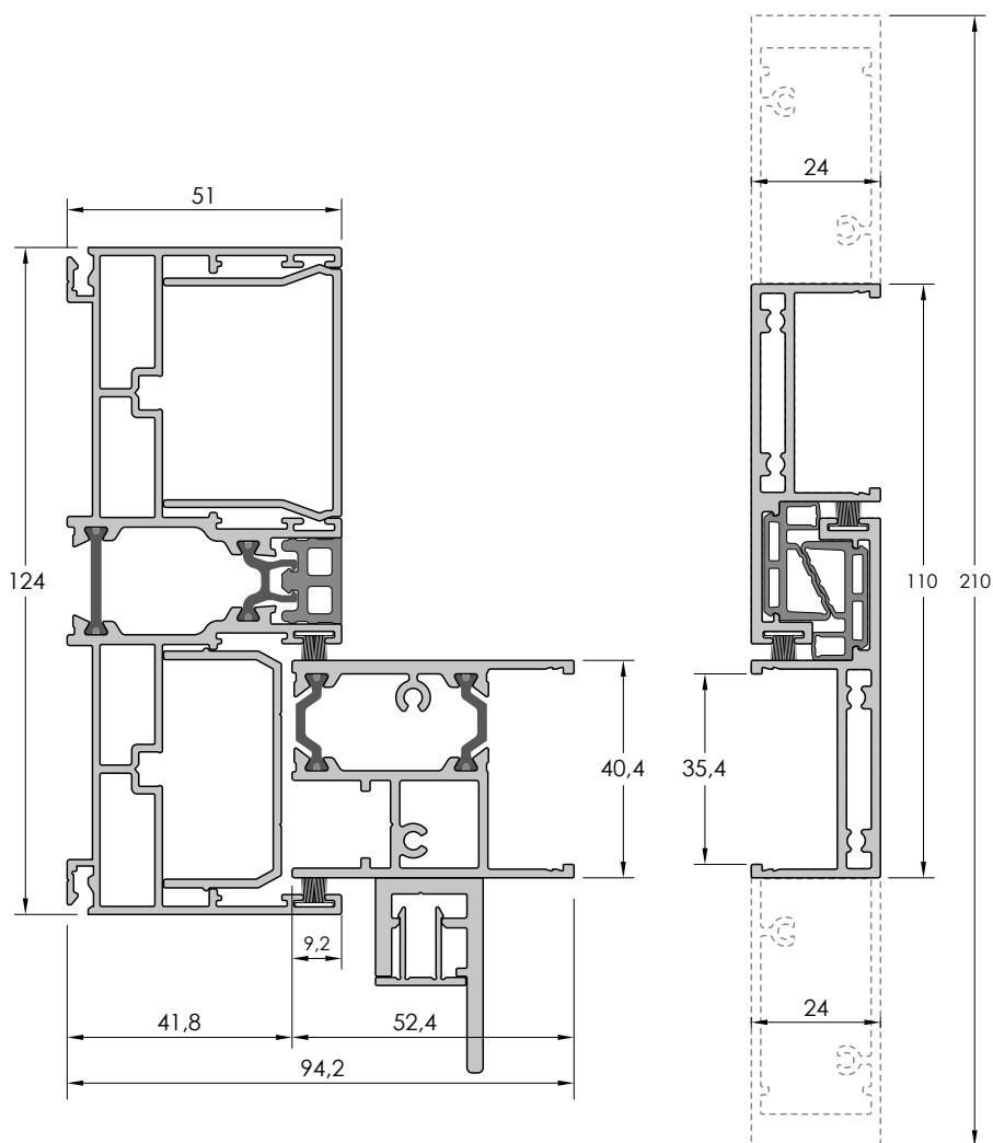
SECCIÓN HORIZONTAL, NUDO LATERAL Y NUDO CENTRAL NORMAL / REFORZADO
