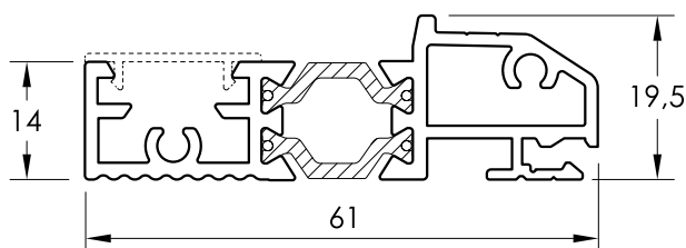
PF 091 UMBRAL PARA CERRADEROS IT-61-NG
