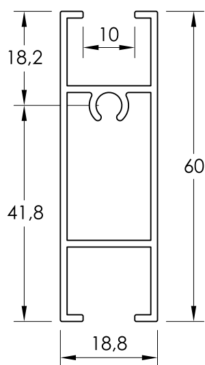
27201 PARTELUCES DE 60
