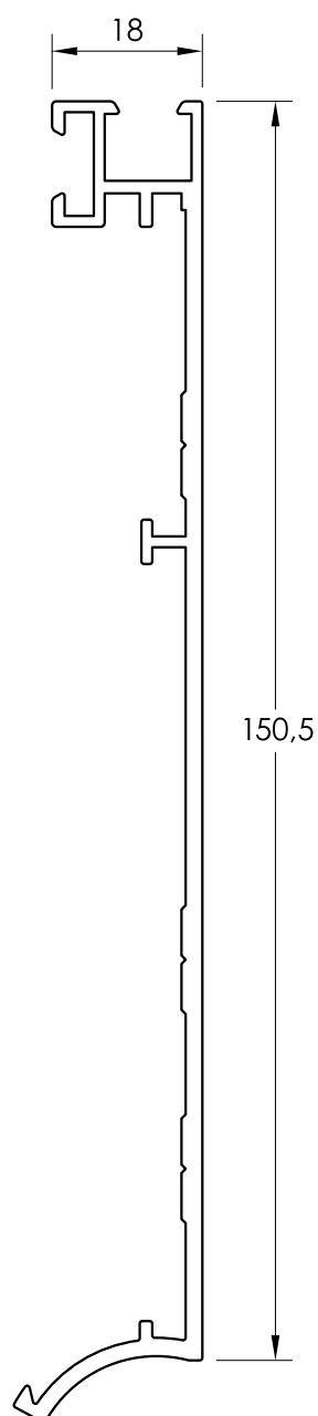
65457 BASCULANTE DE 150
