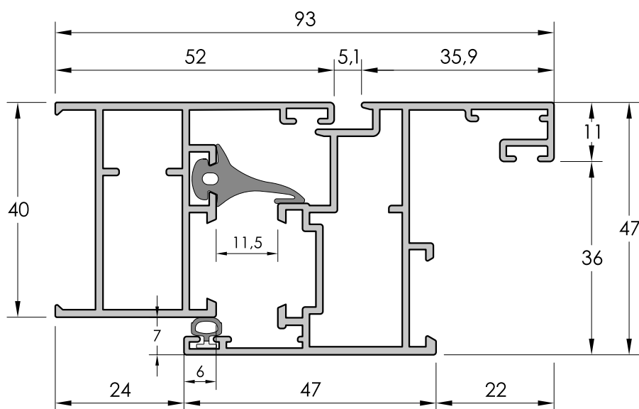
SECCIÓN HORIZONTAL MARCO 34143 - HOJA 35126
