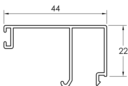
34027 JUNQUILLO DE 44
