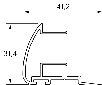
24142 PERFIL DE CRUCE CURVO
