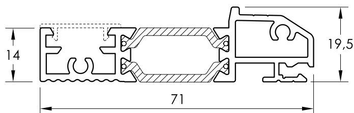
PM 091 UMBRAL IT-71-NG PARA CERRADEROS
