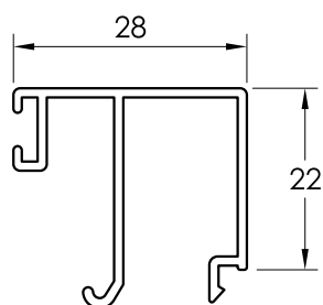
34021 JUNQUILLO DE 28
