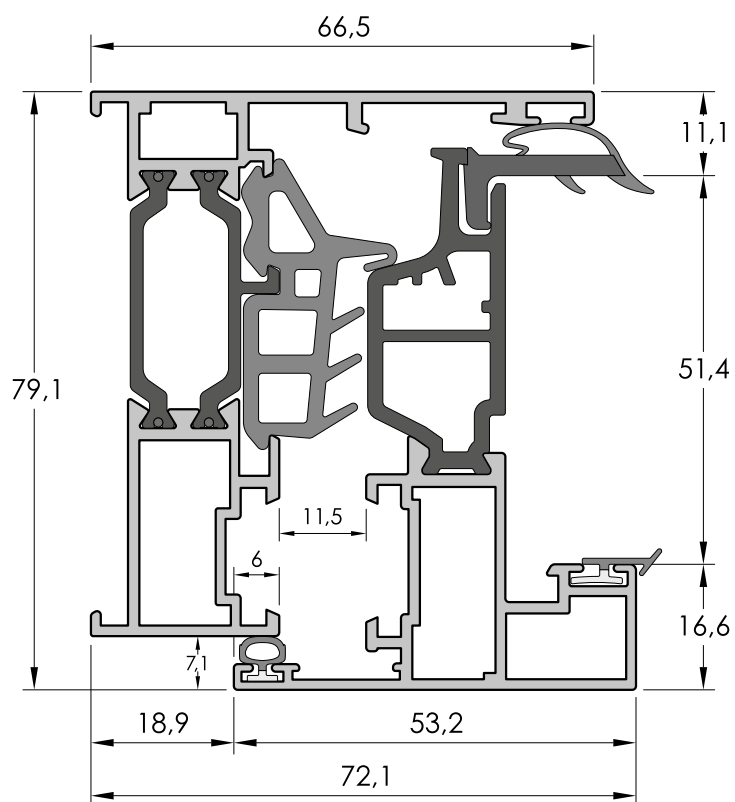
SECCIÓN HORIZONTAL MARCO PL001 - HOJA PL004
