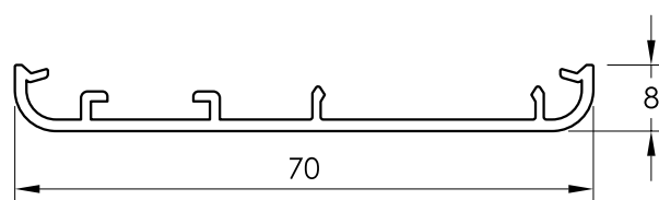
63497 SOLAPA CURVA DE 70 mm.
