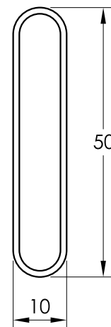
60770 OVALINA 50x10
