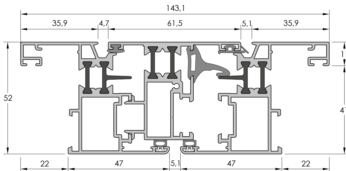
SECCIÓN HORIZONTAL HOJA PA053 - INVERSOR PA055 - HOJA PA053
