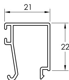
34022 JUNQUILLO DE 21
