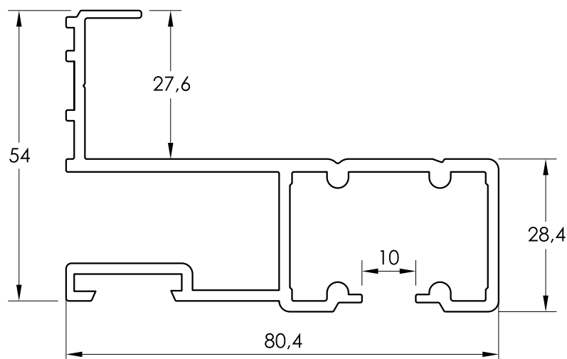
65003 GUÍA SUPERIOR
