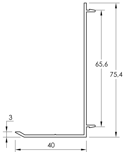
75008 SOLAPA DE 40 mm.
