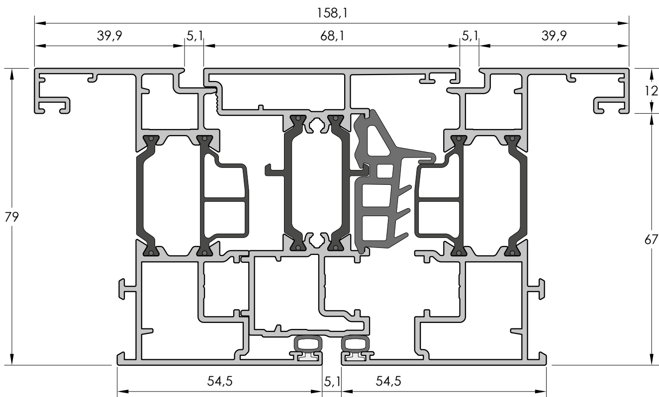
SECCIÓN HORIZONTAL HOJA PM 040 - INVERSOR PM 051 - HOJA PM 040
