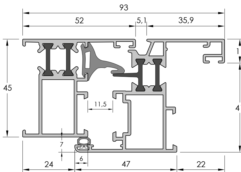
SECCIÓN HORIZONTAL MARCO PA001 - HOJA PA053
