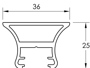
24308 REFUERZO HOJA
