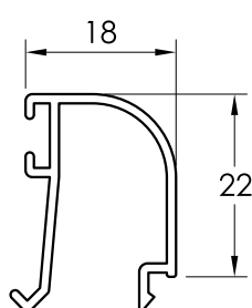
34048 JUNQUILLO DE 18
