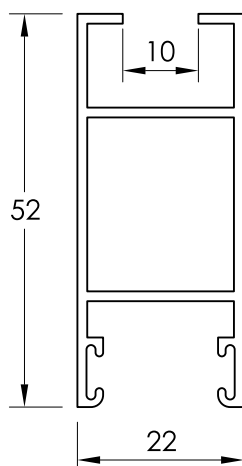
27153 HOJA LATERAL
