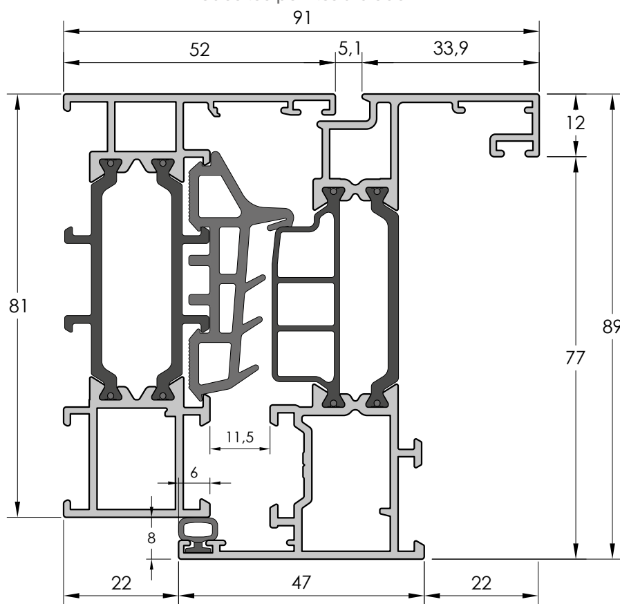
SECCIÓN HORIZONTAL MARCO PS001 - HOJA RECTA PS030
