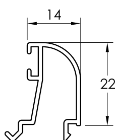
34049 JUNQUILLO DE 14
