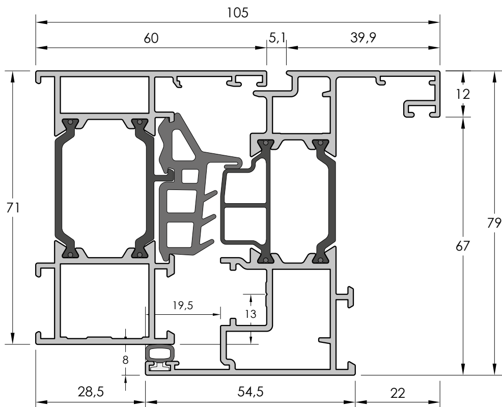
SECCIÓN HORIZONTAL MARCO PM 002 - HOJA PM 040
