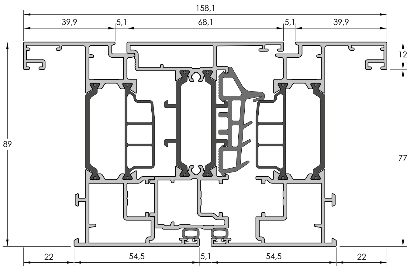
SECCIÓN HORIZONTAL HOJA PS 040 - INVERSOR PS 051 - HOJA PS 040
