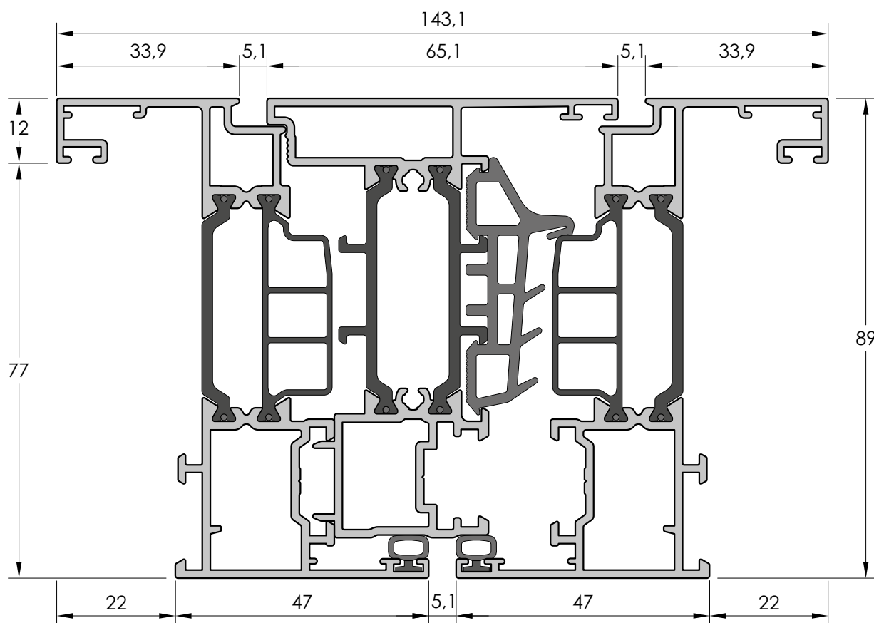
SECCIÓN HORIZONTAL HOJA PS030 - INVERSOR PS050 - HOJA RECTA PS030
