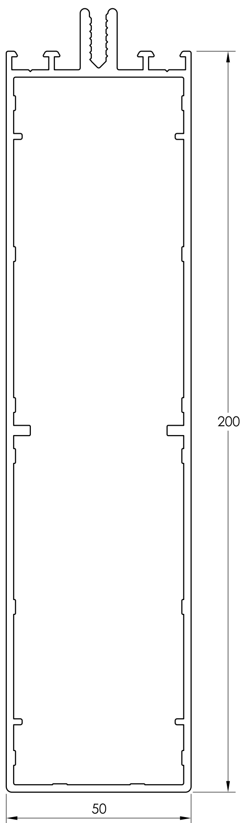
65652 TRAVESAÑO DE 200
