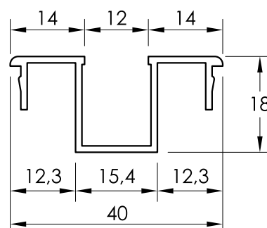
62022 GUÍA DE COMPENSACIÓN
