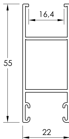
27195 HOJA LATERAL CLIMALIT
