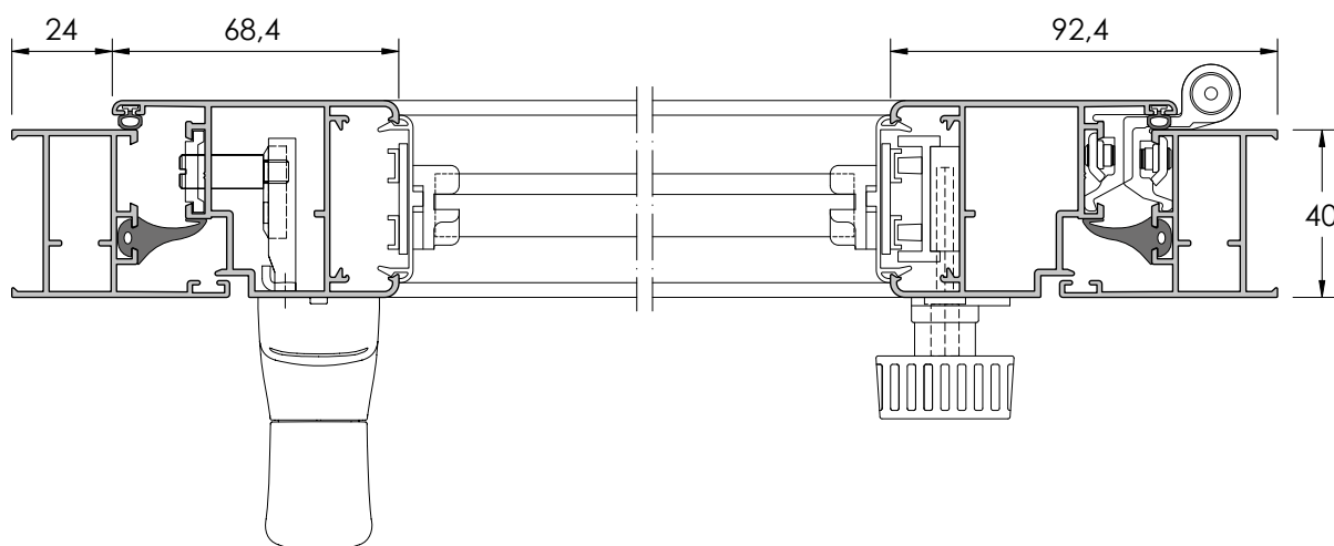
MALLORQUINA C.E. SECCIÓN HORIZONTAL (E: 1/2)
