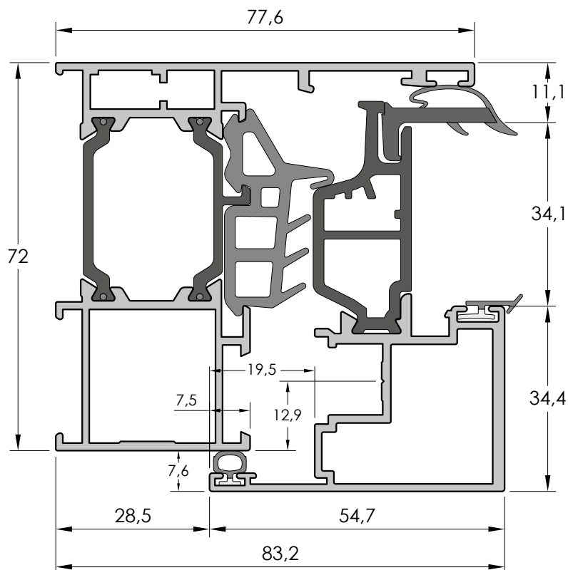
SECCIÓN HORIZONTAL MARCO PL 301 - HOJA PL 086
