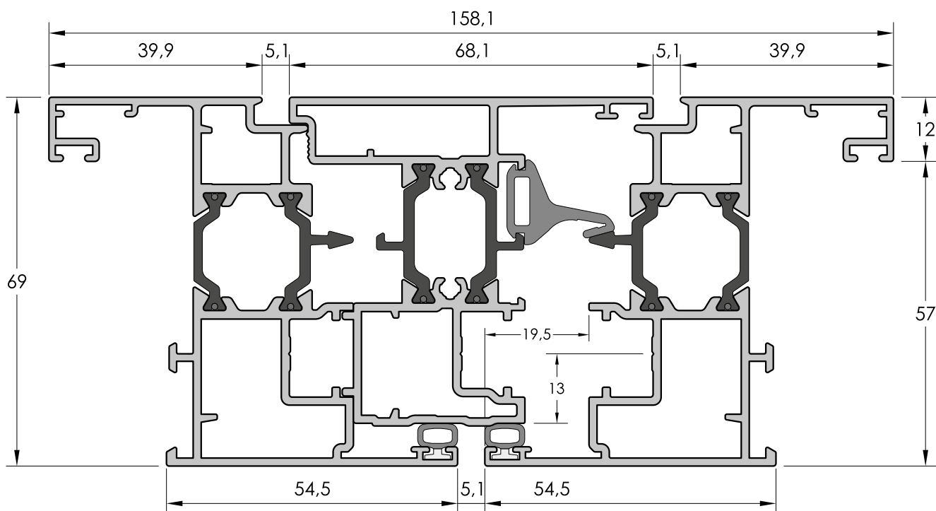
SECCIÓN HORIZONTAL HOJA PF 040 - INVERSOR PF 051 - HOJA PF 040
