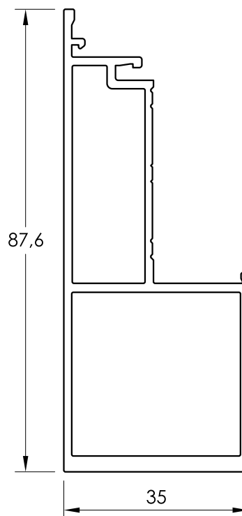
24907 PERFIL DE CRUCE REFORZADO
