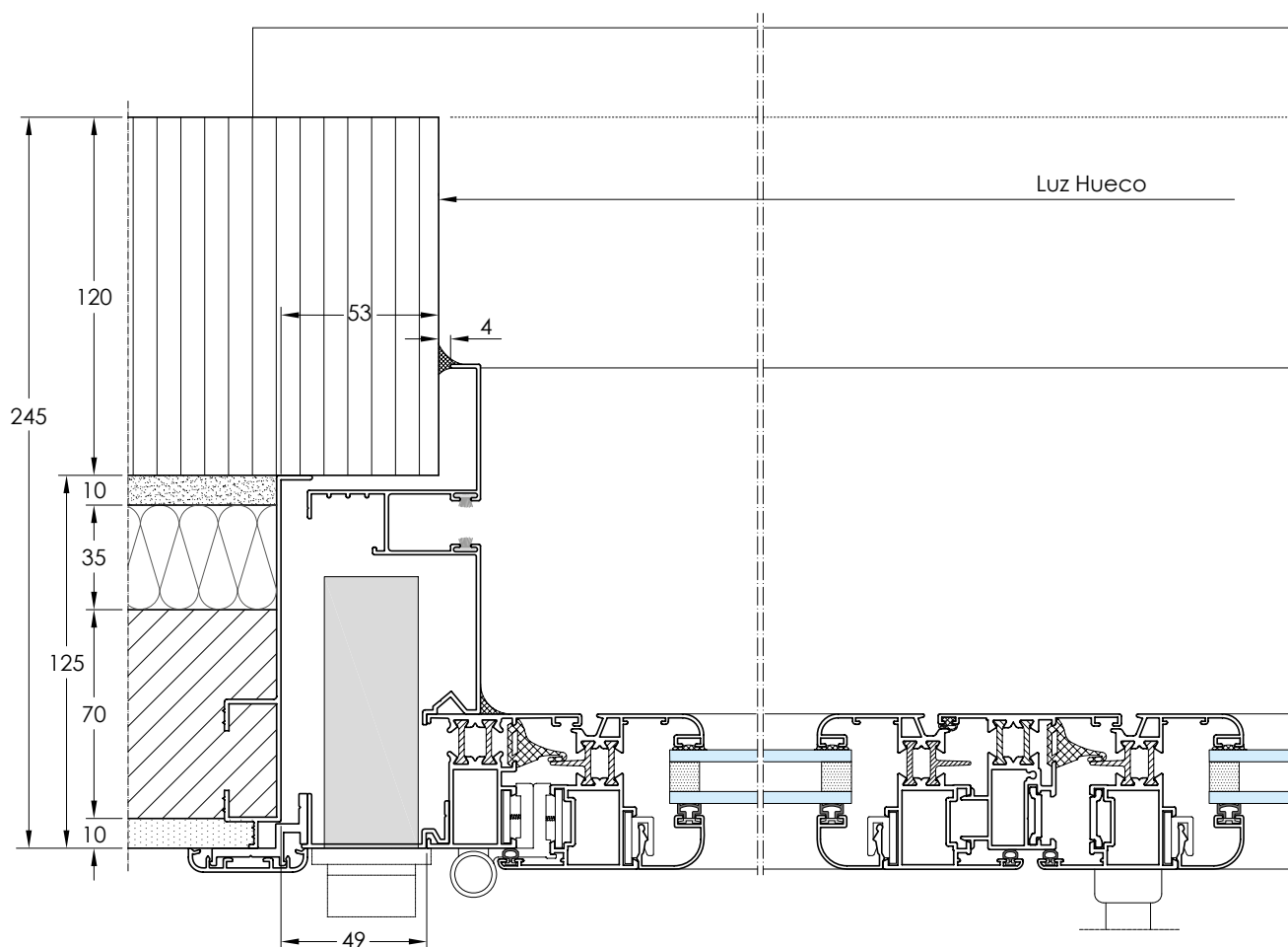
SECCIÓN HORIZONTAL 1-1
