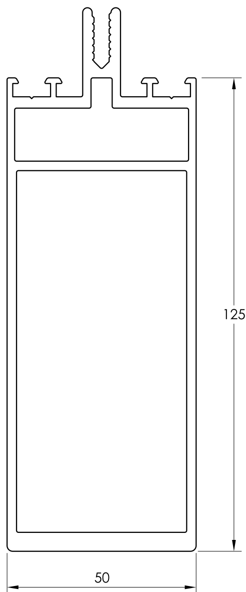
Barras a 6.500 mm. 64399 MONTANTE DE 125
