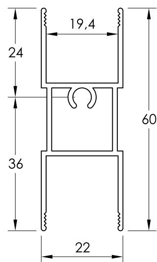
27203 PARTELUCES DE 60 CLIMALIT
