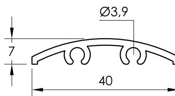
35138 SOLERA PLANA
