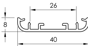
63494 SOLAPA DE 40 mm.
