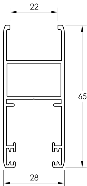
24144 HOJA PERIMETRAL
