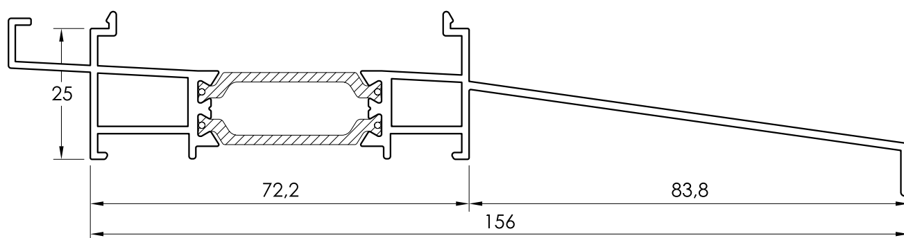
PL 107 CONDENSACIÓN CON ALARGADERA IT-71 RPT
