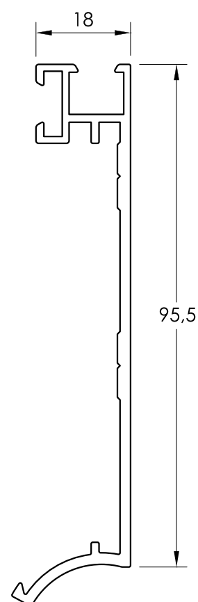
65459 BASCULANTE DE 95
