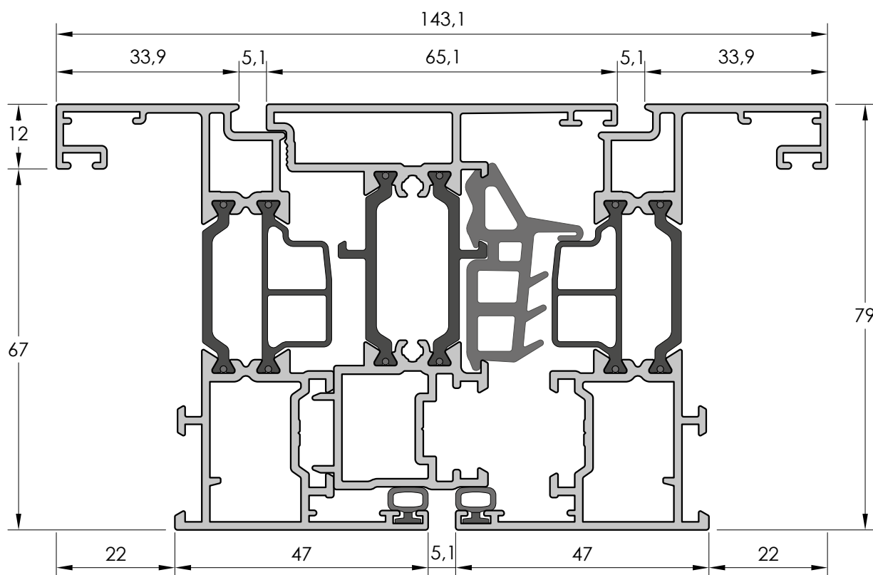
SECCIÓN HORIZONTAL HOJA PM030 - INVERSOR PM050 - HOJA PM030
