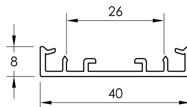
63400 SOLAPA RECTA DE 40 mm.
