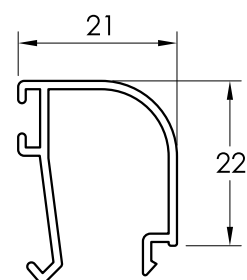
34047 JUNQUILLO DE 21
