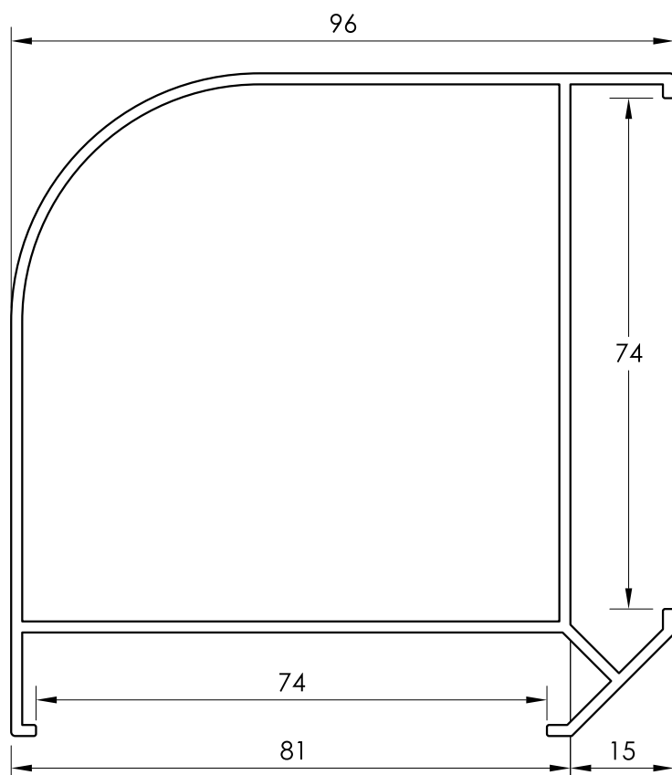
23770 ESQUINERO CURVO
