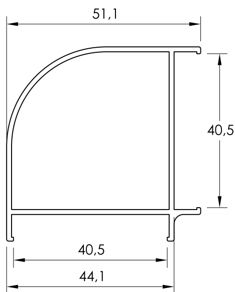
32333 ESQUINERO CURVO 90°
