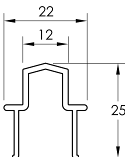
24165 PERFIL 4 HOJAS
