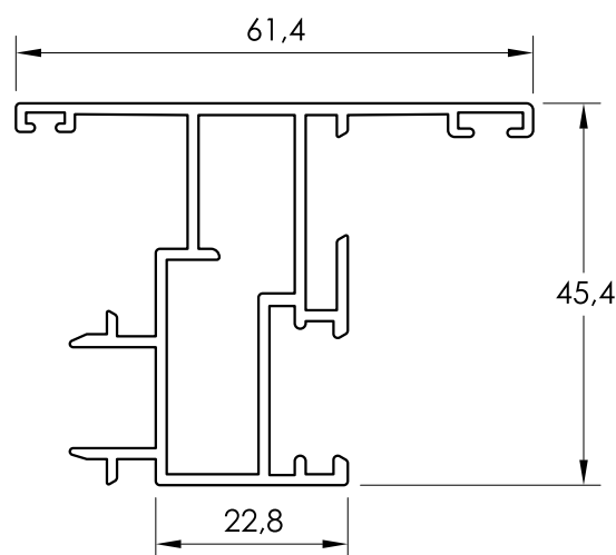
35533 PERFIL INVERSOR
