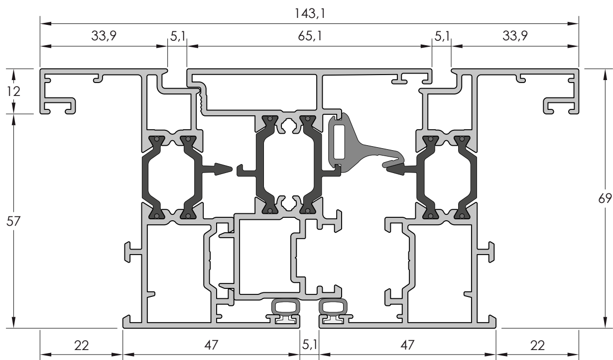
SECCIÓN HORIZONTAL HOJA PF030 - INVERSOR PF050 - HOJA PF030
