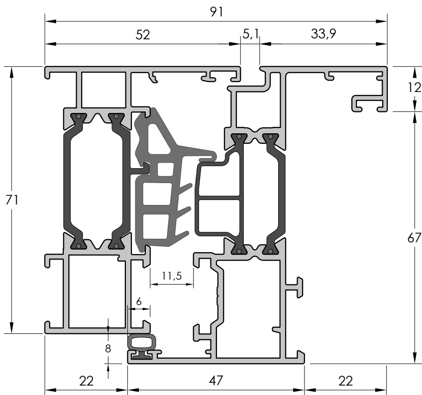
SECCIÓN HORIZONTAL MARCO PM001 - HOJA PM030
