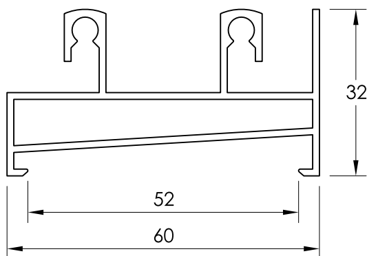
27223 GUÍA INFERIOR TUBULAR
