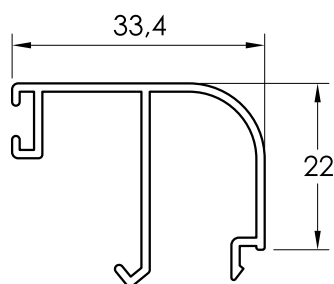
34045 JUNQUILLO DE 33,4
