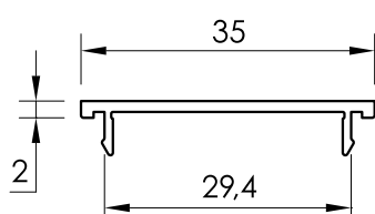
65453 TAPA 35
