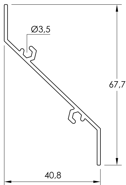
60334 LAMA FIJA
