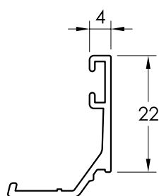
34056 JUNQUILLO DE 4
