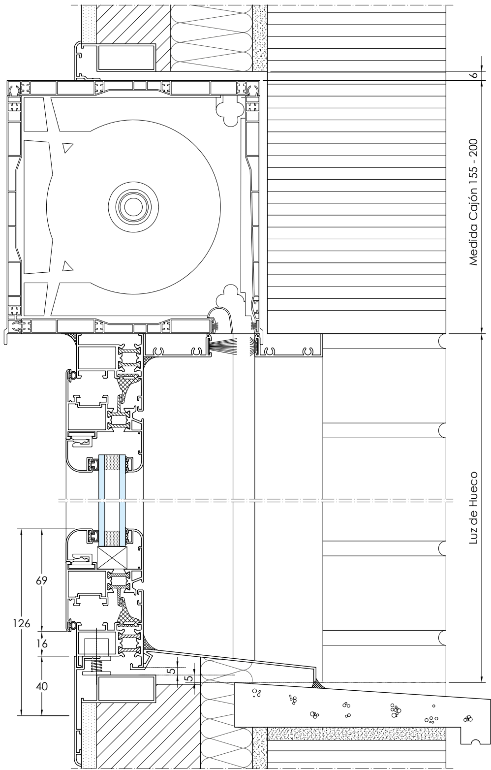
SECCIÓN VERTICAL 2-2
