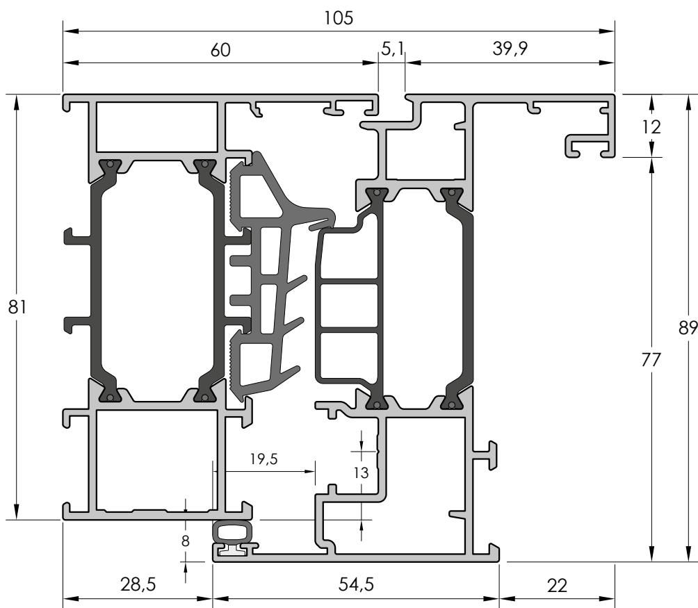
SECCIÓN HORIZONTAL MARCO PS 002 - HOJA PS 040
