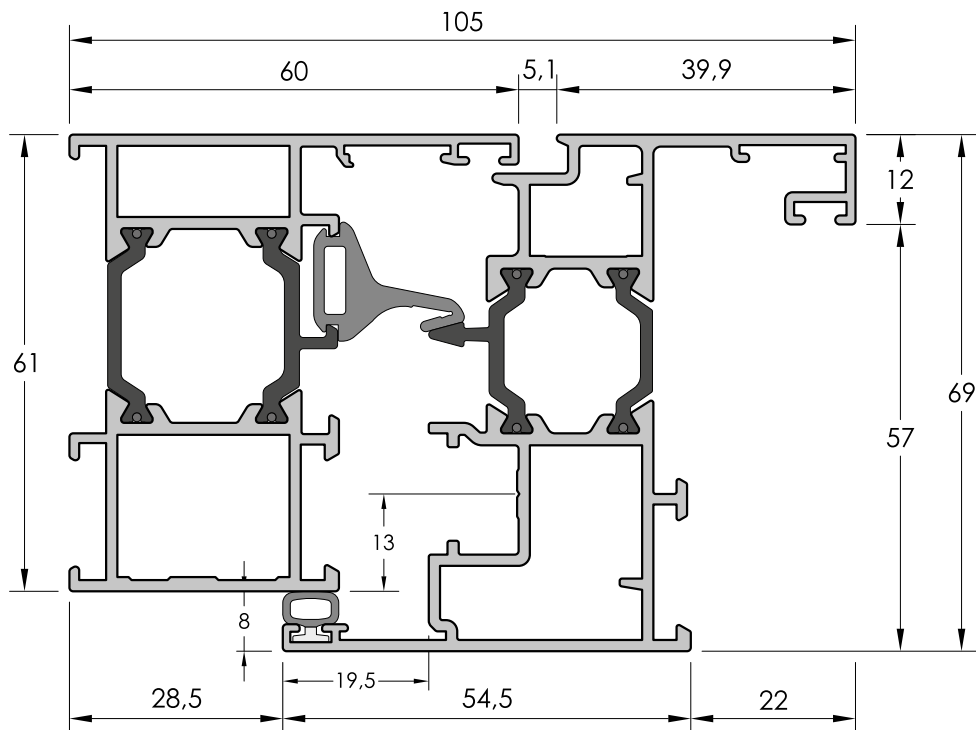
SECCIÓN HORIZONTAL MARCO PF 002 - HOJA PF 040
