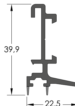
AH 45816 ENGANCHE CENTRAL HOJA + FIJO
