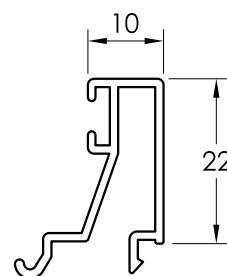
34075 JUNQUILLO DE 10
