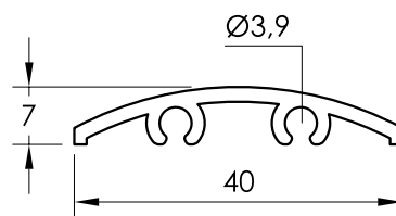
35138 SOLERA PLANA
