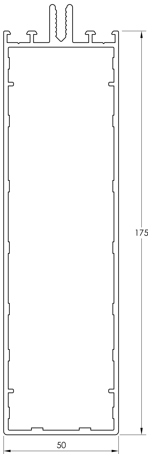
64960 TRAVESAÑO DE 175
