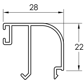
34046 JUNQUILLO DE 28
