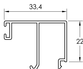
34020 JUNQUILLO DE 33,4
