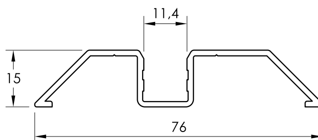
65018 GUÍA INFERIOR SOBRE SUELO
