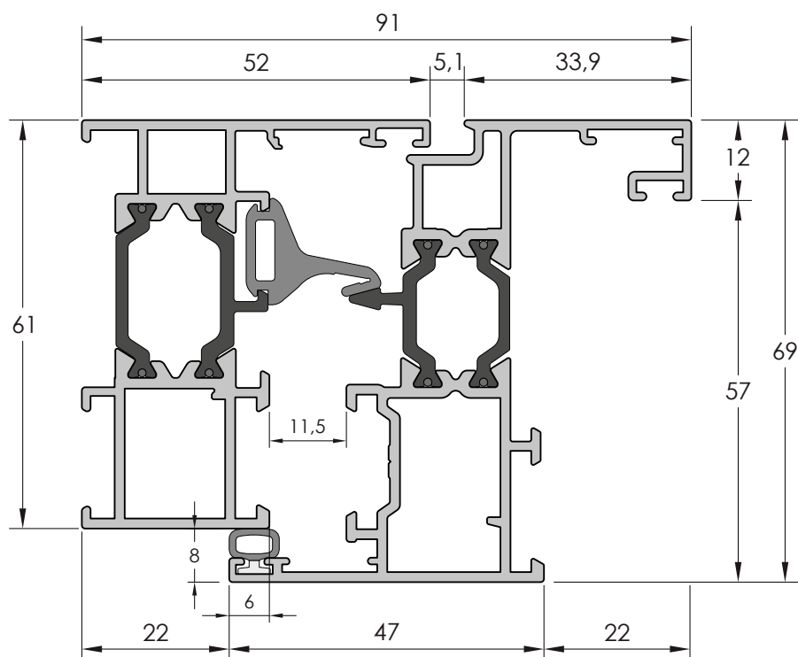
SECCIÓN HORIZONTAL MARCO PF001 - HOJA PF030
