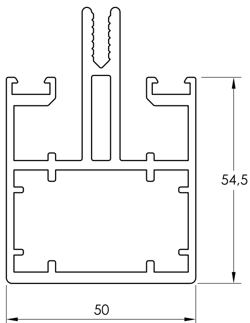
64449 MONTANTE DE 55
