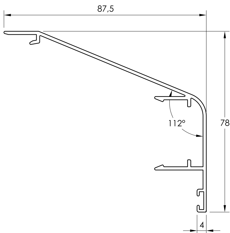
65006 TAPA SUPERIOR
