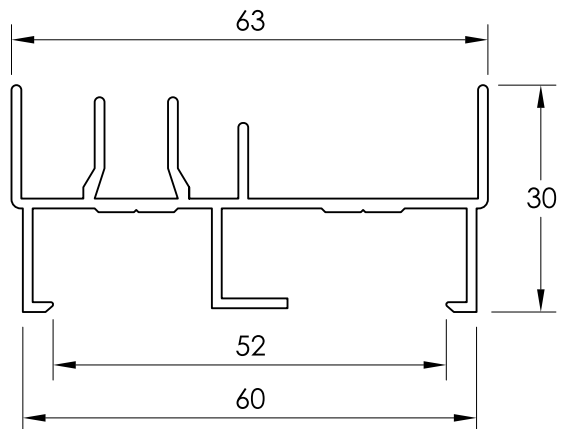
27094 MARCO LATERAL
